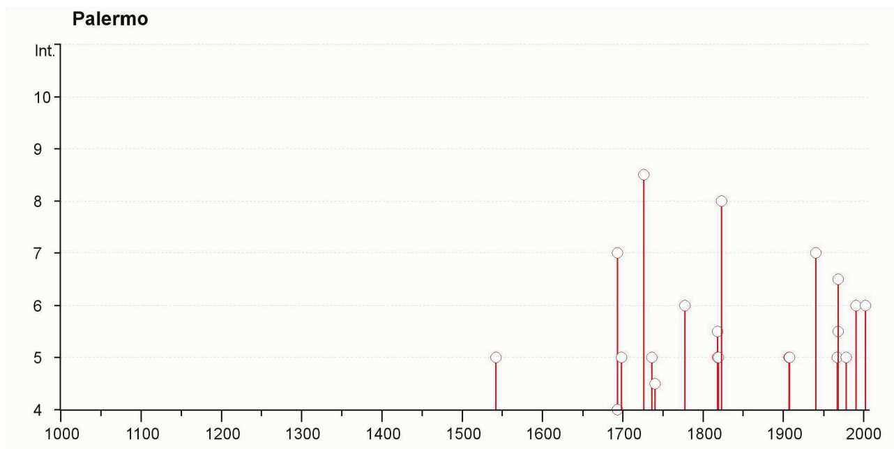
Figura 6a Intensità dei terremoti riportate storicamente nel comune dell'area di discarica di Bellolampo (PA), considerata nel Progetto SIGLOD.
