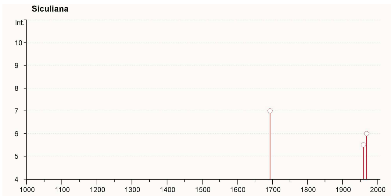
Figura 6b Intensità dei terremoti riportate storicamente nel comune dell'area di discarica di Siculiana (AG), considerata nel Progetto SIGLOD.
