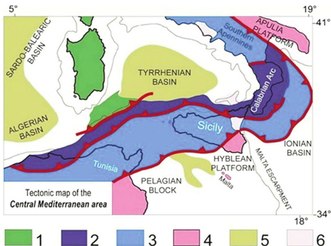
Figura 1 Schema tettonico del Mediterraneo centrale: 1) Corsica-Sardegna; 2) arco Kabilo-Peloritano-Calabro; 3) unità Appenninico-Maghrebidi e dell'avampae deformato; 4) avampae ed avampae poco deformato; 5) aree in estensione; 6) vulcaniti plio-quaternarie [Catalano et al., 1996].
