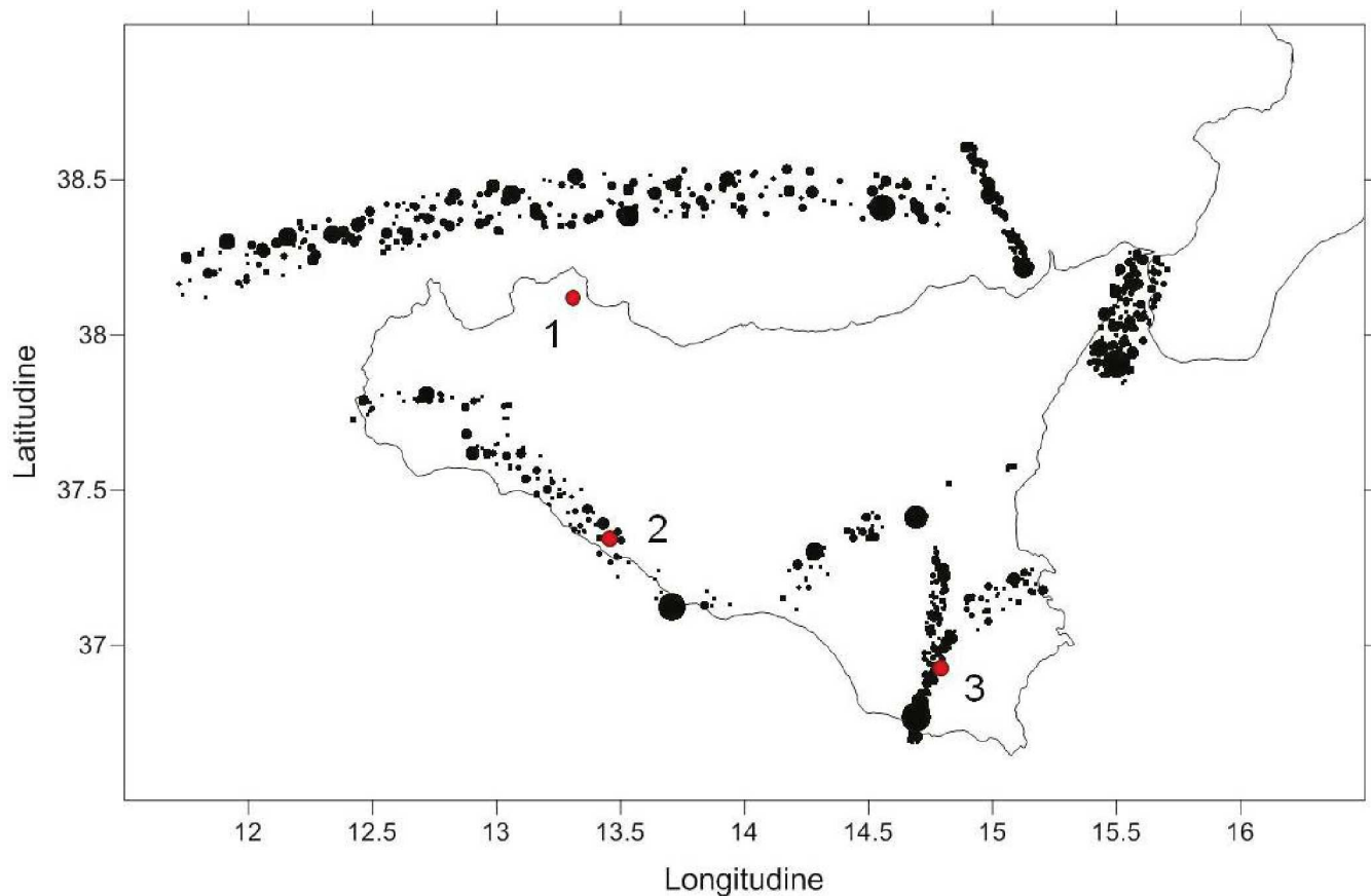
Figura 11 Mappa epicentrale del catalogo sismico sintetico ottenuto per i primi 1000 anni di simulazione sulle principali strutture sismogenetiche riconosciute in Sicilia. Le dimensioni dei simboli neri degli epicentri sono scalate con la magnitudo. I pallini rossi mostrano la posizione dei siti di discarica considerati nello studio: 1 - Bellolampo (PA), 2 - Siculiana (AG), 3 - Cava dei Modicani (RG). Si può notare che i due siti meridionali, Siculiana (AG) e Cava dei Modicani (RG), sono situati praticamente su due strutture sismogenetiche (rispettivamente quelle di Castelvetro-Gela e di Scicli-Giaratana) e pertanto sono i più esposti a effetti da parte di eventi sismici.
